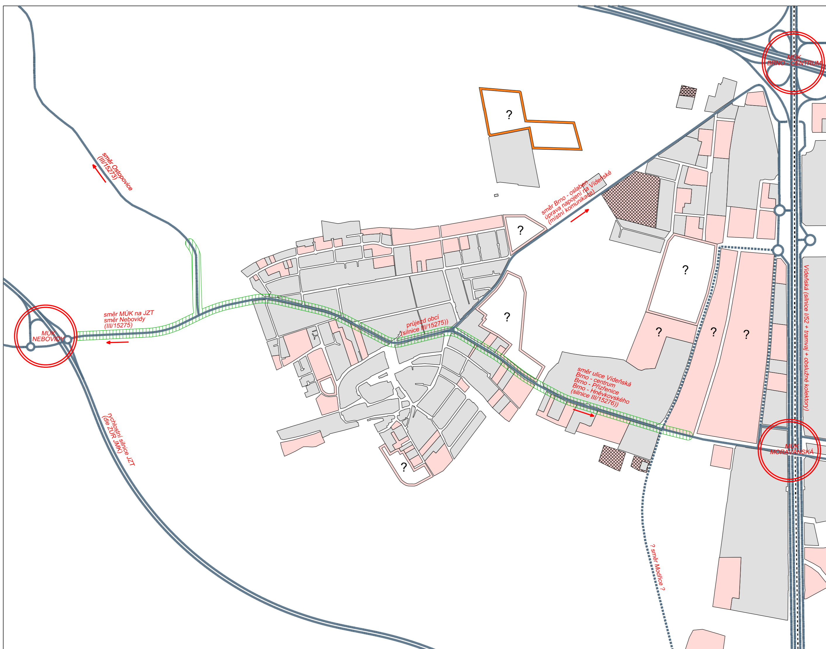
Jihozápadní tangenta (rychlostní silnice I.třídy) dle ZÚR JMK bez doprovodné silniční sítě III. třídy
